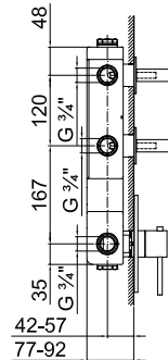
ART. 6002SB Parte esterna / External pieces / Parties externes / Up-Teil / Parte externa
