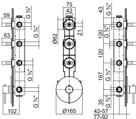
ART. 6003SB Parte esterna / External pieces / Parties externes / Up-Teil / Parte externa
