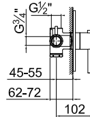
ART. 6000SB Parte esterna / External pieces / Parties externes / Up-Teil / Parte externa
