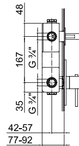
ART. 6001SB Parte esterna / External pieces / Parties externes / Up-Teil / Parte externa
