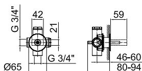
ART. 6090SB Parte esterna / External pieces / Parties externes / Up-Teil / Parte externa
