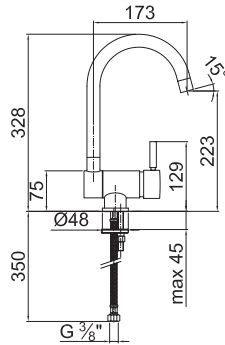
ART. 1859F Miscelatore lavello / Sink mixer / Mitigeur évier / Einhand-Kuchen Mischer / Monomando fregadera
