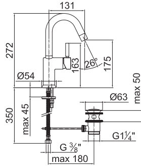
ART. 1804F Gruppo lavabo / Washbasin / Lavabo 1 trous / Waschtischarmatur / Lavabo
