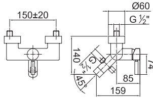
ART. 1818 Vasca esterno / Bath-tub mixer / Bain-douche externe / Aufputz-Wannen / Baño ducha
