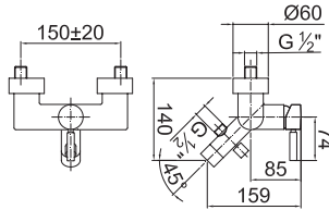
ART. 1815 Vasca esterno / Bath-tub mixer / Bain-douche externe / Aufputz-Wannen / Baño ducha
