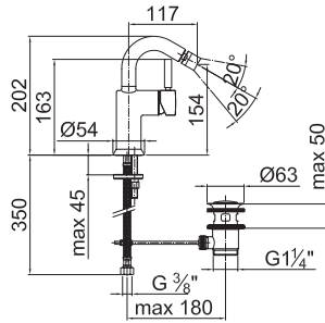
ART. 1808F Miscelatore Bidet / Bidet mixer / Mitigeur bidet / Einhand-Bidet Mischer / Monomando bidè
