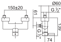
ART. 1826 Doccia esterno / Exposed shower mixer / Douche externe / Aufputz-Brause / Ducha
