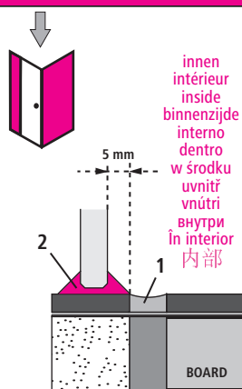
1 Wartungsfuge / Joint de maintenance / Maintenance joint / Voegnaad / Fughe di manutinenze Junta de mantenimiento / Spoina wymagająca konserwacji / Spära pro údržbu / Servisná medzera Технологический шов / Rost pentru lucrări de întreținere / 维护缝
