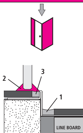
2 Versiegelung / Scellement / Sealing / Siliconen-kitnaad / Sigillatura Sellado / Uszczelnienie zewnętrzne / Uzavirací náter / Tesniaca hmota Герметик / Sigilare / 封闭层
