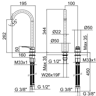
ART. B106WF Batteria lavabo / Washbasin / Lavabo 3 trous / Waschtischarmatur / Lavabo 3 piezas
