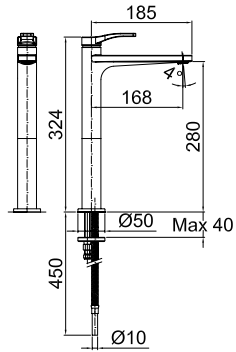
ART. B006WF Gruppo lavabo / Washbasin / Lavabo 1 trous / Waschtischarmatur / Lavabo
