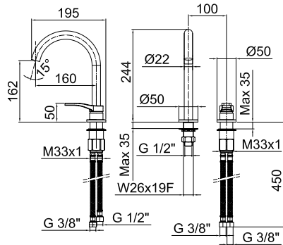
ART. B104WF Batteria lavabo / Washbasin / Lavabo 3 trous / Waschtischarmatur / Lavabo 3 piezas
