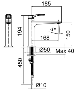
ART. B003WF Gruppo lavabo / Washbasin / Lavabo 1 trous / Waschtischarmatur / Lavabo
