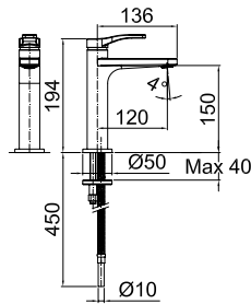
ART. B004WF Gruppo lavabo / Washbasin / Lavabo 1 trous / Waschtischarmatur / Lavabo
