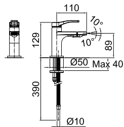
ART. B008WF Bidet monoforo / 1 hole bidet / Mélangeur bidet / Einlochbidet / Monobloc bidé
